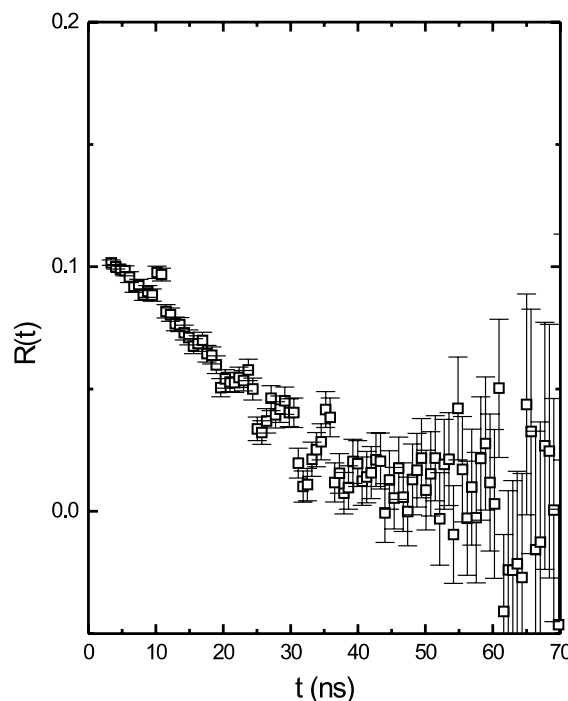
Figura 2. Espectro temporal R(t) en función del tiempo, medido a 1200K.
