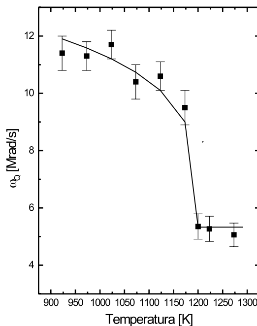
Figura 4. La frecuencia cuadripolar \omega_Q en función de la temperatura T.
